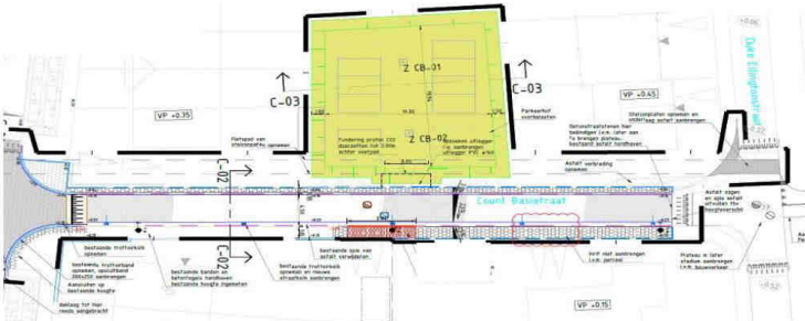
Figuur 3 : Inrichtingstekening van Jazzroute tot Duke Ellingtonstraat
